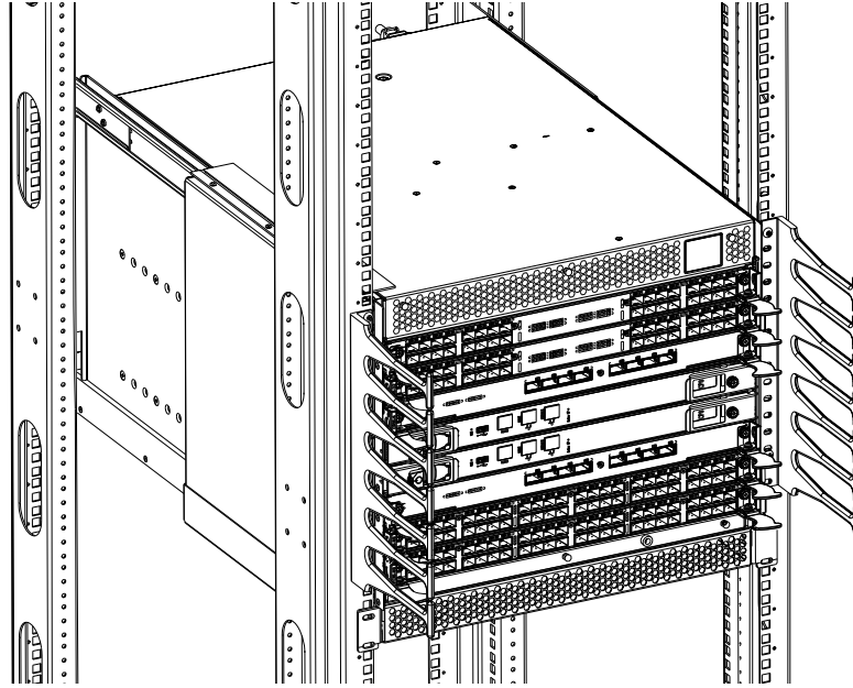
ŞEKİL 5 Dikey kablo düzenleme parmak aksamı
